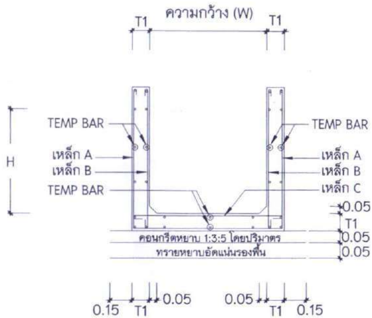
รายละเอียดเหล็กเสริมวาง คสล. มาตราส่วน No scale
